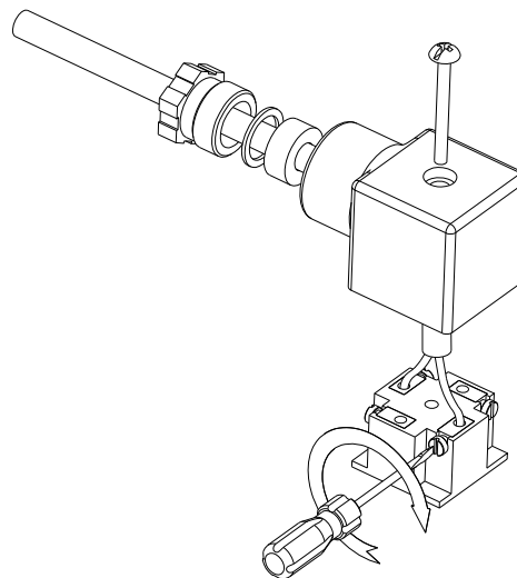
Figura 2 – Conexión de los cables
